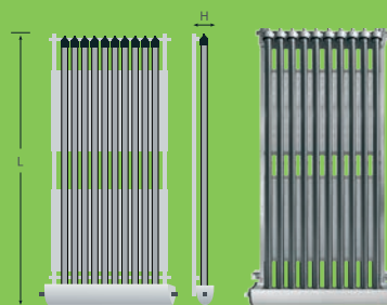
Panel solarny 10-rurowy SCL-SRP 10
